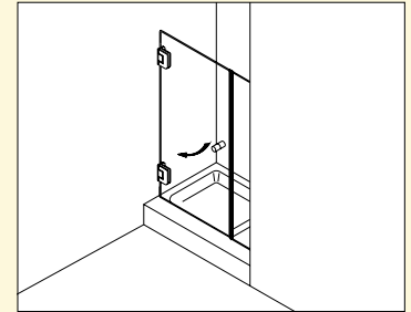
Typ / Type 110 Nischenkabine, 1 Drehtür, 1 Fixteil
