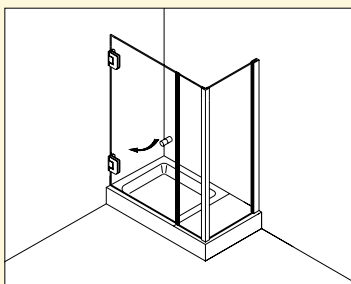
Typ / Type 140 Eckkabine, 1 Drehtür, 1 Fixteil, 1 Seitenwand
