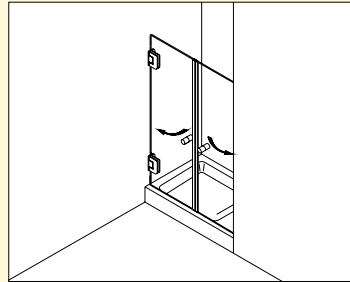
Typ / Type 105 Nischenkabine, 2 Drehtüren
