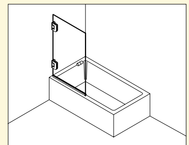
Typ / Type 170 Eckkabine, 1 Drehtür auf Badewanne
