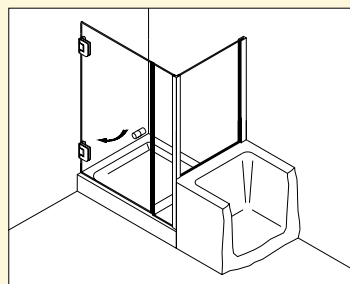
Typ / Type 141 Eckkabine, 1 Drehtür, 1 Fixteil, 1 verkürzte Seitenwand
